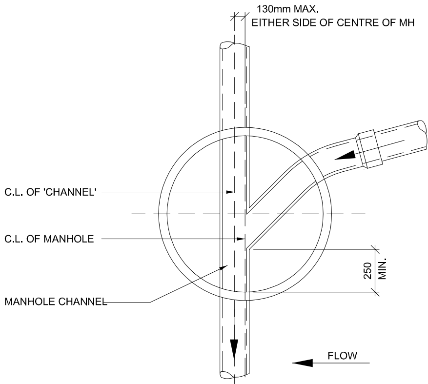
MANHOLE - PLAN VIEW N.T.S.
