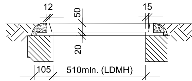
MANHOLE FRAME SECTION
